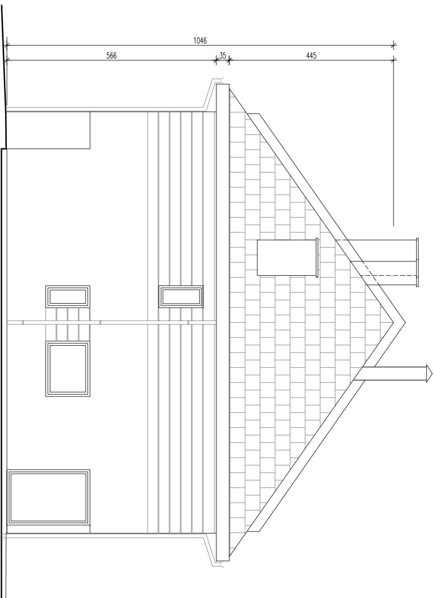
ELEWACJA PÓŁNOCNA - BUDYNEK B
