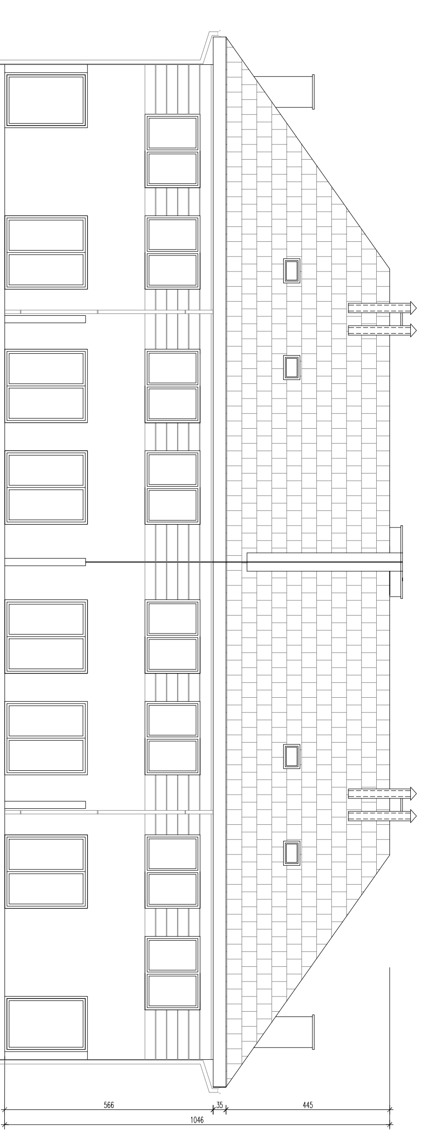
ELEWACJA PÓŁNOCNO-ZACHODNIA - BUDYNEK A, B
