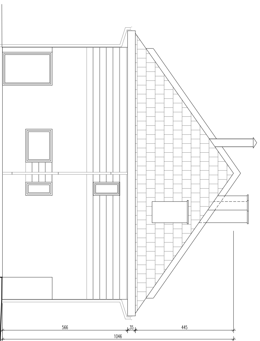
ELEWACJA POŁUDNIOWA - BUDYNEK A
